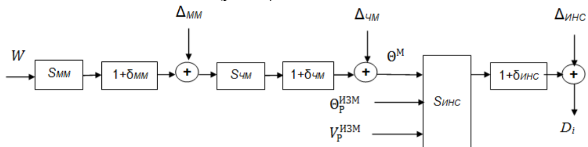
Рисунок 5 – Структурная модель канала с ИИС для классификации термограмм
